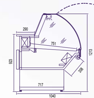
Vista lateral / Side view / Vue latérale / Vista de lado
