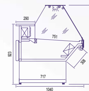
Vidros Rectos / Straight Glats Vitres Droits / Vidrios Retos
